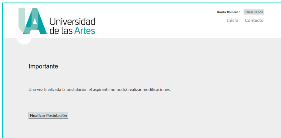
Figura 9 – Finalizar Postulación
